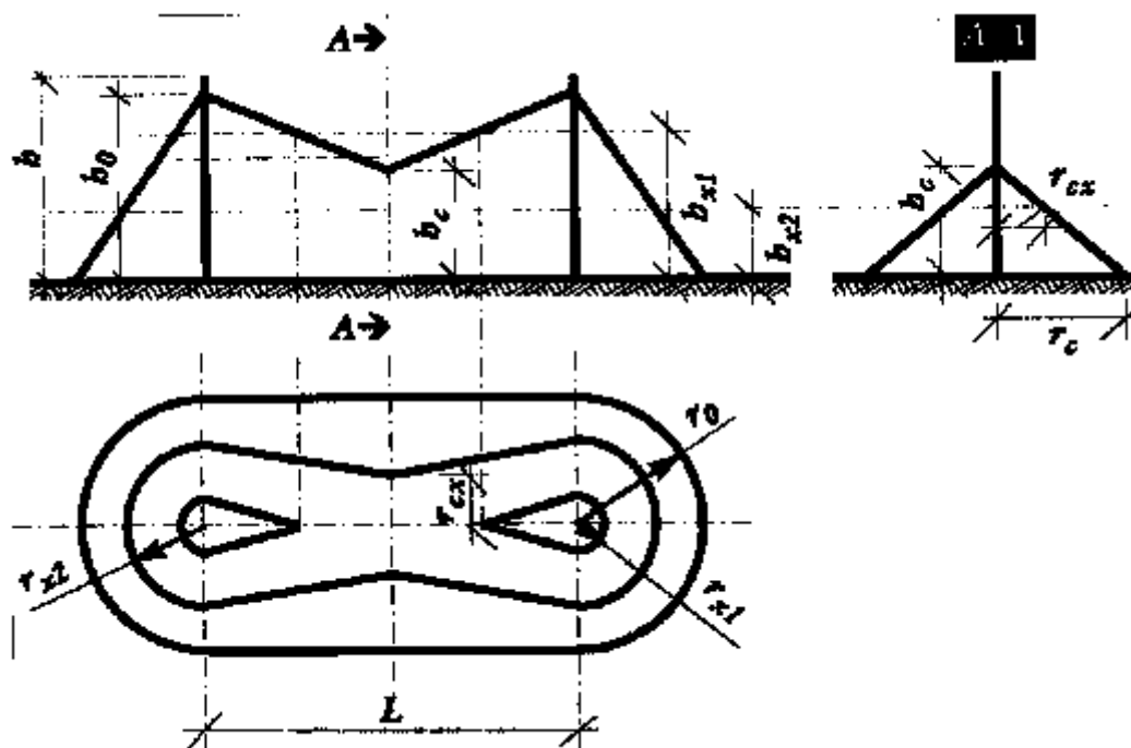
Фиг. 8. Мълниезащитна зона на два прътови мълниеотвода с равни височини до 150 м: L—разстояние между мълниеотводите; h—височина на мълниеотводите; h0—височина на мълниезащитните конуси; r0—радиус на мълниезащитните конуси на нивото на терена; rx1—радиус на мълниезащитния конус на височина hx1; rx2—радиус на мълниезащитния конус на височина hx2; hc—минимална височина на мълниезащитната зона; rc—размер на мълниезащитната зона на нивото на терена, съответстващ на hc; rcx—размер на мълниезащитната зона на височина hx
