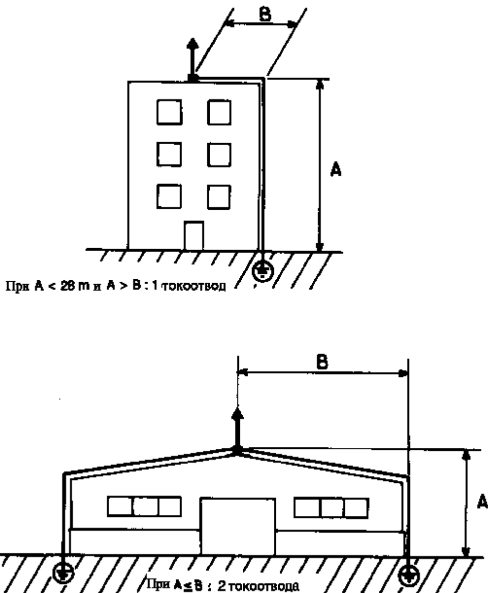
Фиг. 17. Брой на токоотводите
