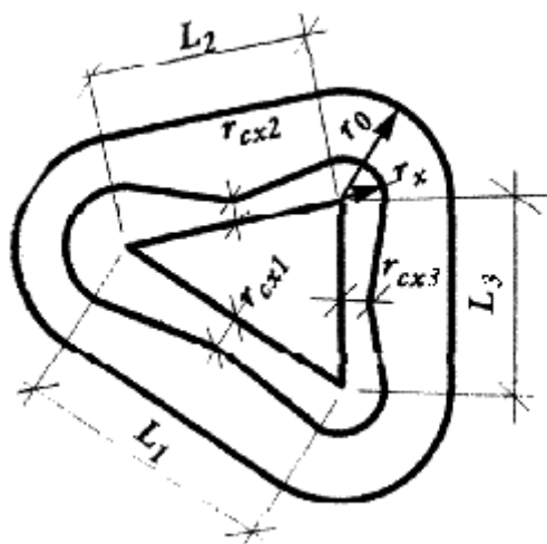
Фиг.10. Мълниезащитна зона на три прътови мълниеотвода с равни височини до 150 m: L1, L2 и L3—разстояния между мълниеотводите; rсх1, rсх2 и rсх3—размери на мълниезащитната зона на височина hx; r0—радиус на защитния конус на нивото на терена; rx—радиус на мълниезащитната зона на височина hx
