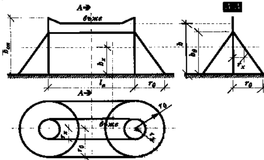
Фиг. 11. Мълниезащитна зона на единично мълниеотводно въже на височина до 150 m: l_a —разстояние между опорите; h_{оп} —височина на опорите; h —отстояние на въжето от терена в зоната на най-големия провес; h_0 —височина на мълниезащитната зона; r_0 —размер на мълниезащитната зона на нивото на терена; r_x —размер на мълниезащитната зона на височина h_x
