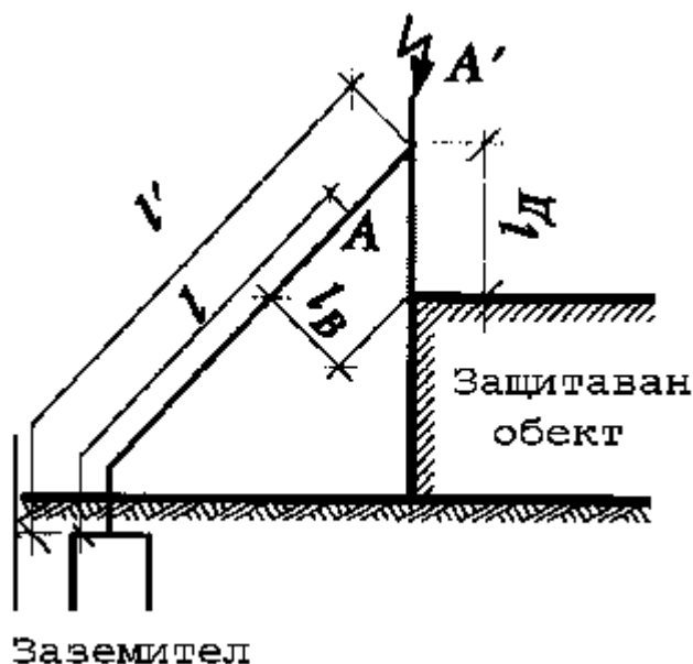
Фиг. 2. Мълниезащита чрез прътов мълниеотвод, изолиран от защитавания обект: А (А')—точка от мълниеотвода, отстояща на минимално разстояние от защитавания обект; l ( l' )—разчетна дължина на мълниеотвода; l_B —минимално разстояние по въздуха между мълниеотвода и защитавания обект; l_D —минимална дължина на електроизолационната опора на мълниеотвода
