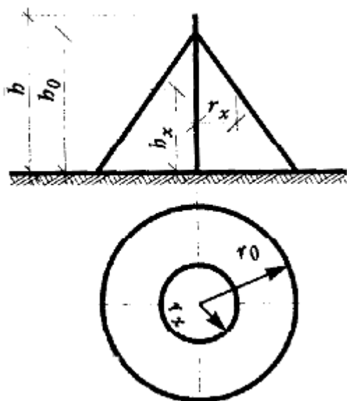
Фиг. 7. Мълниезащитна зона на единичен прътов мълниеотвод с височина до 150 m: h –височина на мълниеотвода; h_0 –височина на мълниезащитния конус; r_0 –радиус на мълниезащитния конус на нивото на терена;
