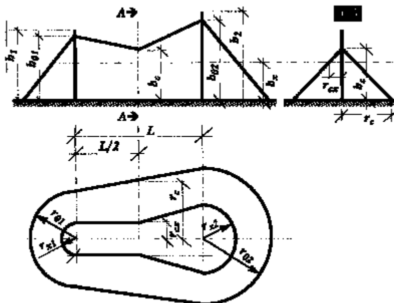
Фиг. 9. Мълниезащитна зона на два прътови мълниеотвода с различни височини до 150 m: L—разстояние между мълниеотводите; h1 и h2—височини на мълниеотводите; h01 и h02—височини на мълниезащитните конуси; r01 и r02—радиуси на мълниезащитните конуси на нивото на терена; rx1 и rx2—радиуси на мълниезащитните конуси на височина hx; hc—минимална височина на мълниезащитната зона; rс—размер на мълниезащитната зона на нивото на терена, съответстващ на hc; rсх—размер на мълниезащитната зона на височина hx
