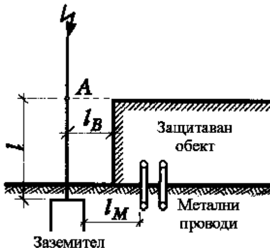
Фиг. 1. Мълниезащита чрез отделностоящ прътов мълниеотвод: А—точка от мълниеотвода, съответстваща на най-високата част на защитавания обект; l —разчетна дължина на мълниеотвода; l_{в} —минимално разстояние по въздуха между мълниеотвода и защитавания обект; l_{м} —минимално разстояние между заземителя и подземните метални проводни
