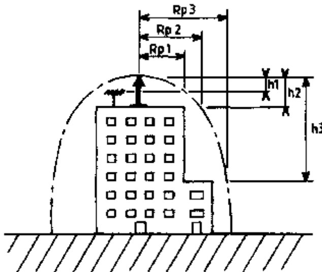
Фиг. 15. Радиуси на защита: h_p е височина на върха на мълниеприемника с изпреварващо действие по отношение на хоризонтална повърхност, преминаваща през върха на разглеждания защитаван обект; R_{p1} —радиус на защита на мълниеприемника с изпреварващо действие за разглежданата височина
