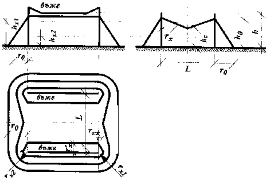
Фиг. 12. Мълниезащитна зона на две успоредни мълниеотводни въжета на височина до 150 m: L —разстояние между мълниеотводните въжета; h —отстояние на въжетата от терена в зоната на най-големия провес; h_0 —височина на мълниезащитната зона; r_0 —размер на мълниезащитната зона на нивото на терена; r_{x1} и r_{x2} —радиуси на мълниезащитната зона на височина h_{x1} и h_{x2} ; r_{cx} —размер на мълниезащитната зона на височина h_{x2} ; r'_x —размер на мълниезащитната зона на височина h_{x1} ; h_c —минимална височина на мълниезащитната зона
