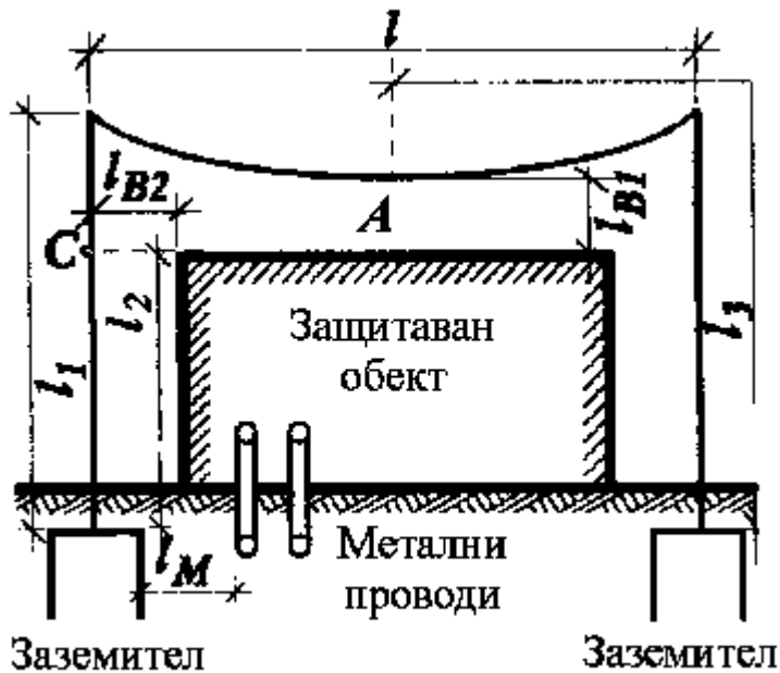
Фиг. 4. Мълниезащита чрез мълниеотводно въже, разположено на височина до 150 m: А–точка от мълниеотводното въже, отстояща на минимално разстояние от защитавания обект; С–точка от опората на мълние от водното въже, отстояща на минимално разстояние от защитавания обект; l–разстояние между опорите на мълниеотводното въже; l1–височина на опорите на мълниеотводното въже; l2–разчетна височина на опората на мълниеотводното въже; l3–разчетна дължина на мълниеотвода; lB1–минимално разстояние по въздуха между мълниеотводното въже и защитавания обект; lB2–минимално разстояние по въздуха между опората на мълниеотводното въже и защитавания обект; lM–минимално разстояние между заземителя и металните подземни проводни
