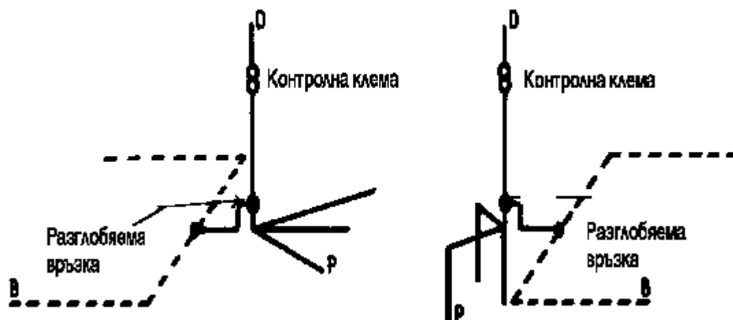
Фиг. 13. Типови решения на заземители: D - токоотвод; В - контур в основата на сградата; P - заземител за мълниезащитата
